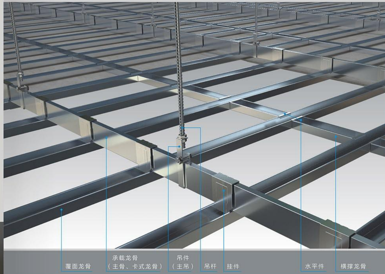
主龙骨与副龙骨的组合
