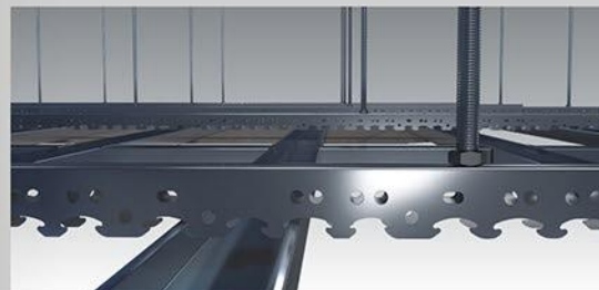
卡式龙骨与副龙骨的组合
